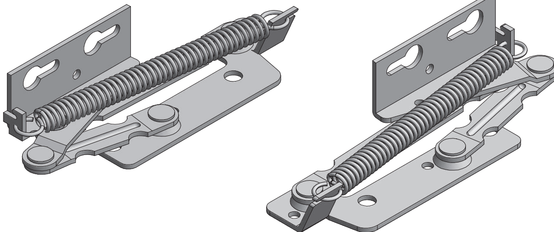
1. Zawias JUNIOR 75° Hinge JUNIOR 75° Петля JUNIOR 75°
