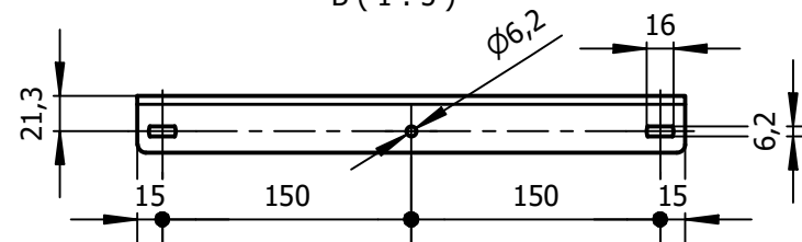
B ( 1 : 5 )
