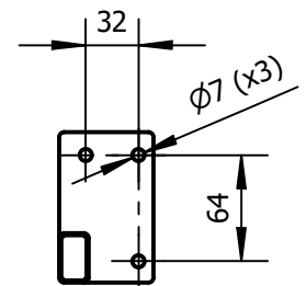
A-A ( 1 : 5 )
